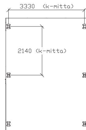
Pohjakuva
